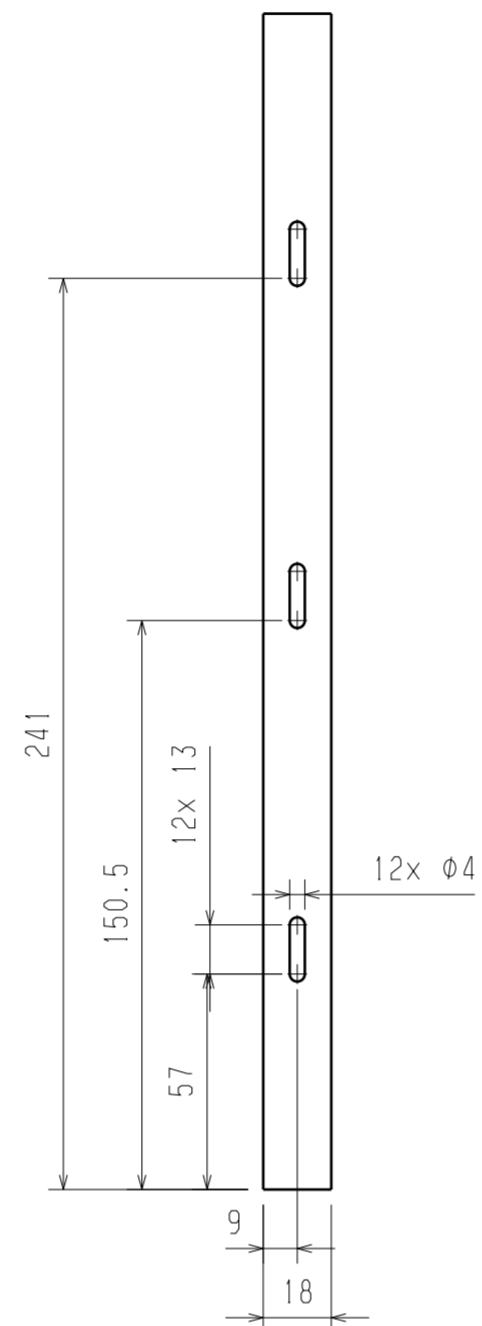
Left view Scale: 1:2
